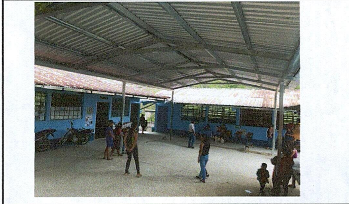
Foto 2: Mejoramiento de patio con Estructura portante a metalica (tipo portico) mas lamina troquelada calibre 26 para reuniones y actividades
